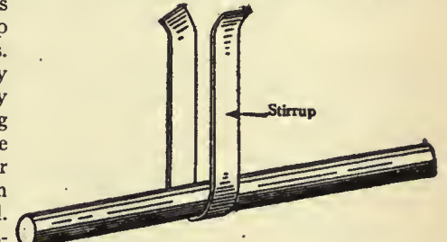
FIG. 14.—Stirrup (Hennebique System).
